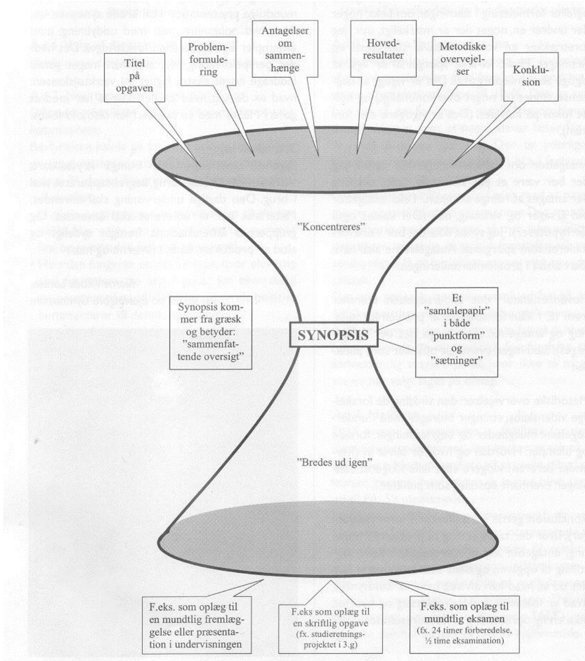
Figur 1: Synopsens opbygning
